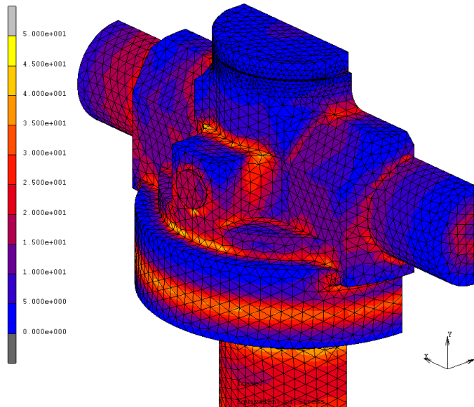
Abbildung 2 Verteilung der Vergleichsspannungen infolge Innendrucks
