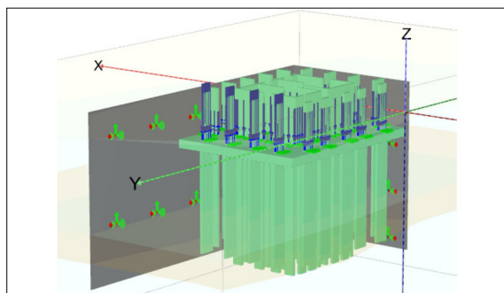
Modell kombinierte Pfahl-Plattenfundation, Plaxis 3D
