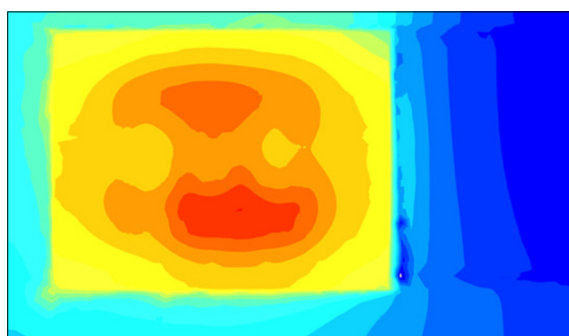
Setzungen, gelb Fundation (gelb = 7 mm, orange = 10 mm, rot = 12 mm)
