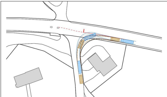
Abbildung 2: Schleppkurve Rechtseinbieger
