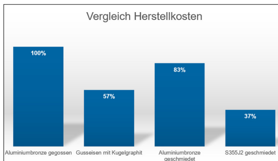
Analyse verschiedener Herstellverfahren
