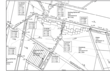
Ausschnitt Entwässerungsplan
